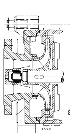
Entrada axial en tamaños \geq 65
