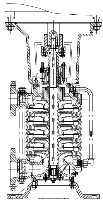
Ejecución V rodamiento V separado en la linterna del motor, a partir del tamaño 100
