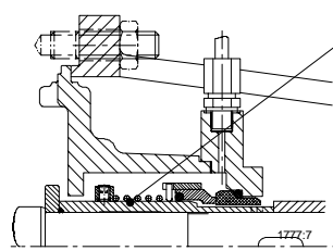
Cierre mecánico sencillo
